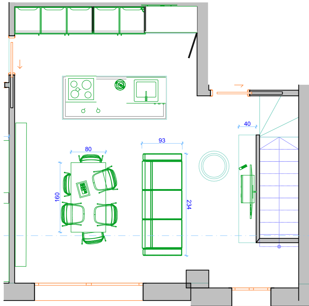
zona giorno versione 1 scala 1:50@A3
